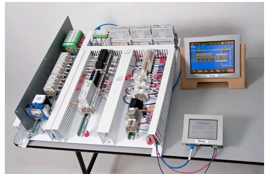
Drop-in subplate
